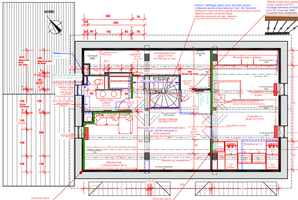
PROJET - COMBLES RÉAMÉNGÉ
