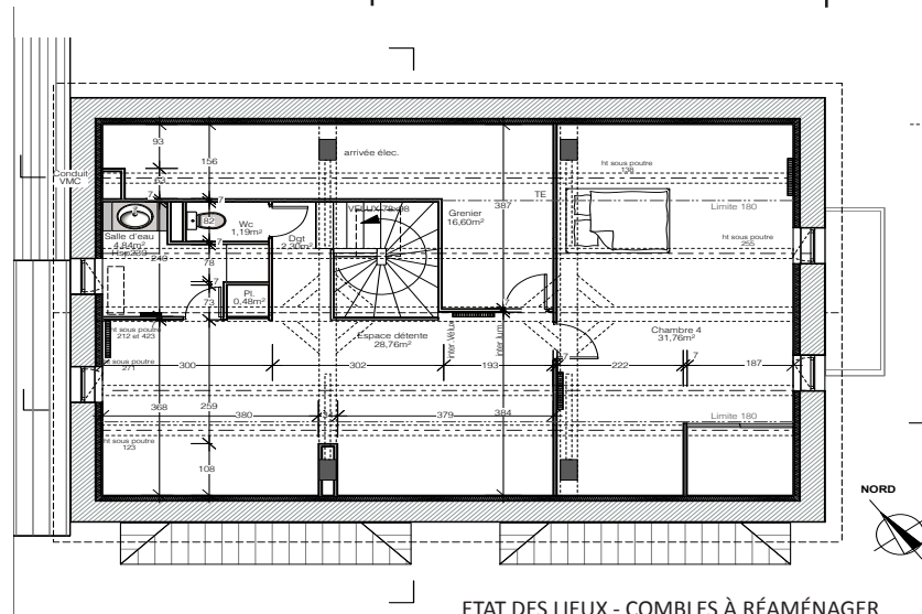
ETAT DES LIEUX - COMBLES À RÉAMÉNGER
